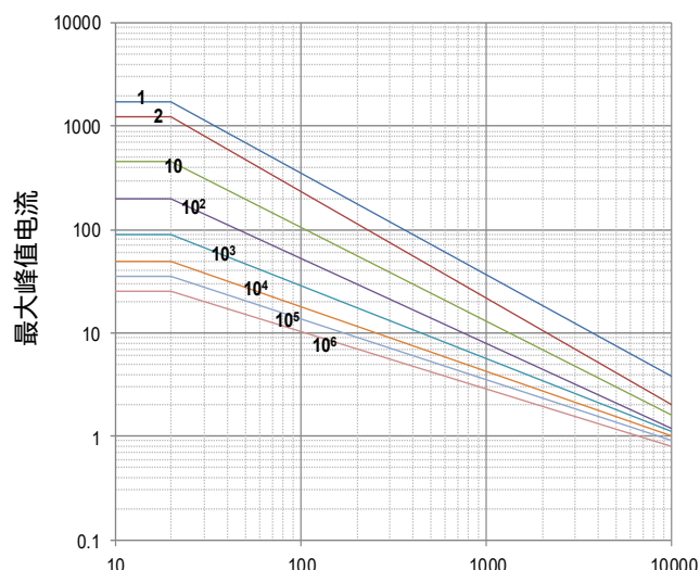
脉冲持续时间 (μs) SFV7D820K to SFV7D821K
